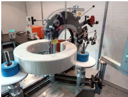
Obrázek 15 Orbitální ovinovačka
